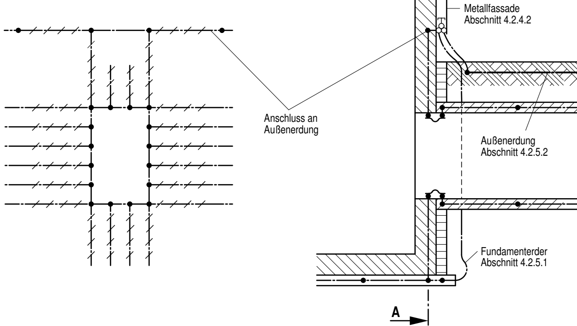
Bild 4-6: Kabelkanal, Verbindung der Kanalabschirmung mit der Metallfassade und dem Fundamenterder bei isoliertem Fundament
