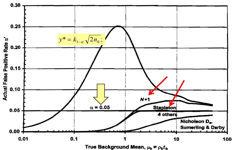
Bild 2-4: Darstellung der tatsächlichen Wahrscheinlichkeit für falsch positive Ergebnisse ( \alpha' ) nach Storm et al für \alpha = 0,05 für verschiedene Berechnungsmodelle als Funktion der Nulleffektimpulszahl.
