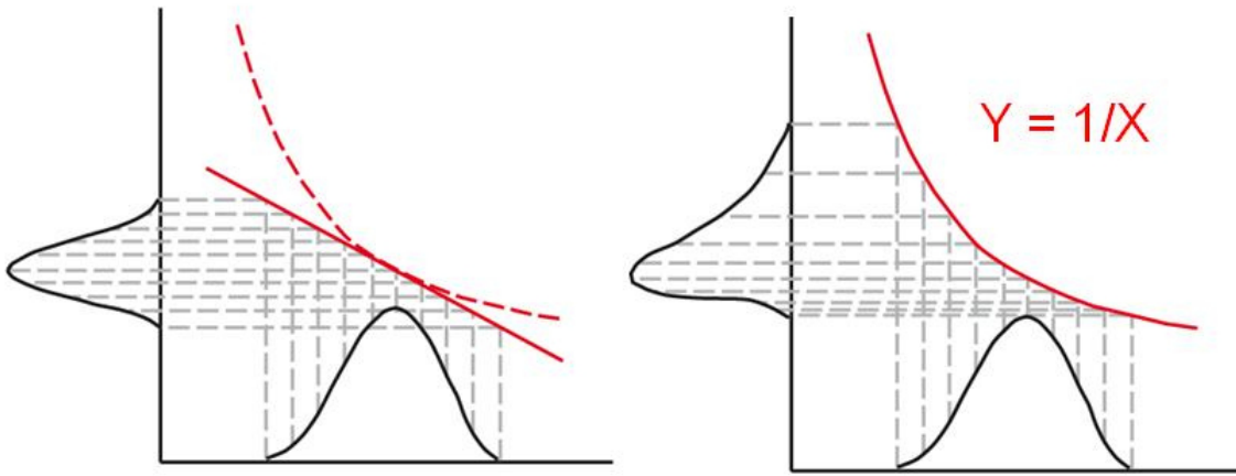
Bild 2-6: Eine normalverteilte Eingangsgröße x wird durch die lineare Approximation am Maximum der Verteilung (Gauß'sche Fehlerfortpflanzung) zu einer normalverteilten Ausgangsgröße y abgebildet (linkes Diagramm). In der Realität führt das Modell der Auswertung y = 1/x zu einer asymmetrischen WDF der Ergebnisgröße y (rechtes Diagramm).
