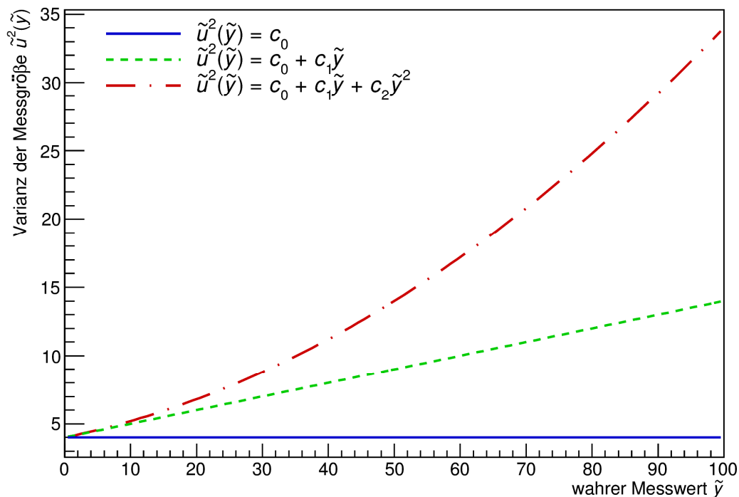
Bild 2-1: Darstellung der Varianz der Messgröße als Funktion des wahren Wertes aufgetragen über den wahren Wert der Messgröße entsprechend den Koeffizienten in den Gleichungen (2-11) bis (2-16). Frühere Regeln zur Bestimmung von Erkennungs- und Nachweisgrenzen führen zu \tilde{u}^2(\tilde{y}) = \text{const} , da implizit c_1 = c_2 = 0 unterstellt worden ist. Dies war nicht korrekt.
