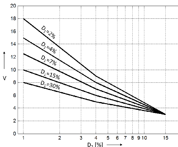
Bild 4-2: Ermittlung des Spektrüberhöhungsfaktors
