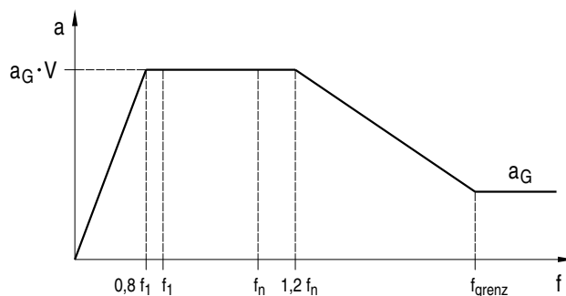
Bild 4-1: Ermittlung der Form des Antwortspektrums
