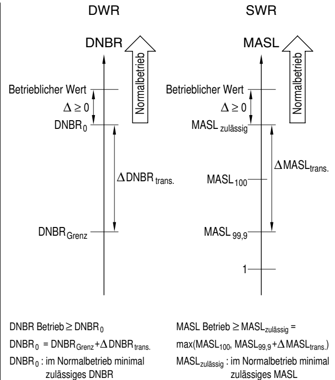
Bild 5-2: Schematische Darstellung der Beziehungen zwischen DNBR- oder MASL-Werten des normalen und anomalen Betriebs
