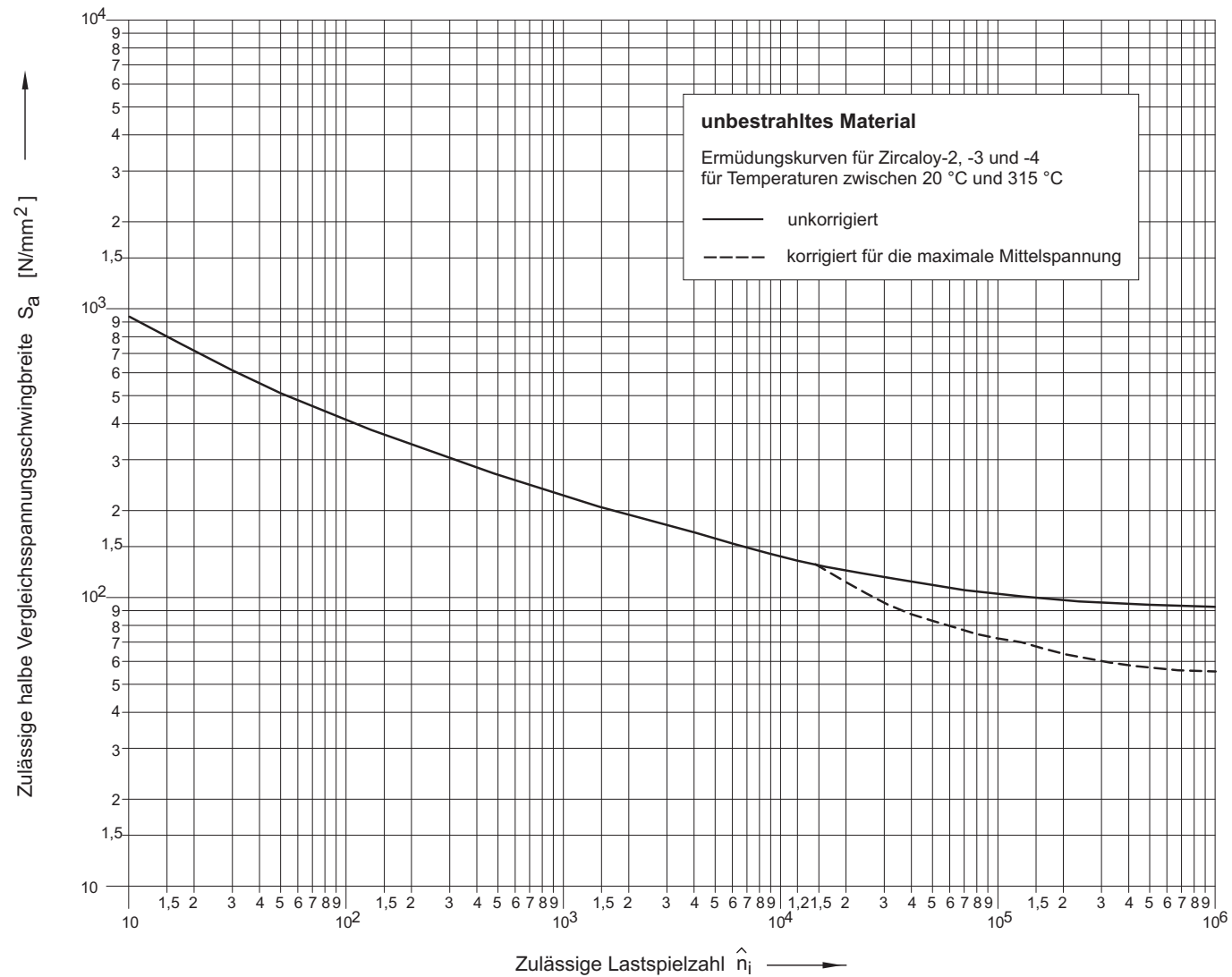
Bild B 5-4: Ermüdungskurven für unbestrahltes Zircaloy- 2, 3 und 4 für Temperaturen zwischen 20 °C und 315 °C
