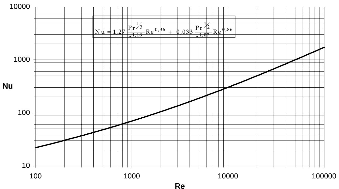
Bild 3-1: Nusselt-Zahl als Funktion der Reynolds-Zahl für \epsilon = 0,39 und Pr = 0,7
