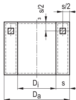
Bild 20-1: Beispiele für Probenentnahmeorte
