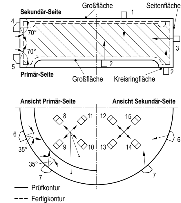
Bild 6-2: Einschallrichtungen 1 bis 15 bei der Ultraschallprüfung geschmiedeter Platten für Rohrböden
