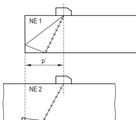
Bild B-15: Schallfeldgeometrien bei der Umwandlung von Transversalwellen
