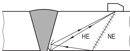
Bild B-16: Prüfung von Komponenten mit Nennwanddicken größer als 8 mm und gleich oder kleiner als 20 mm mittels Longitudinalwellen (Prüfkopf 70 Grad SEL)
