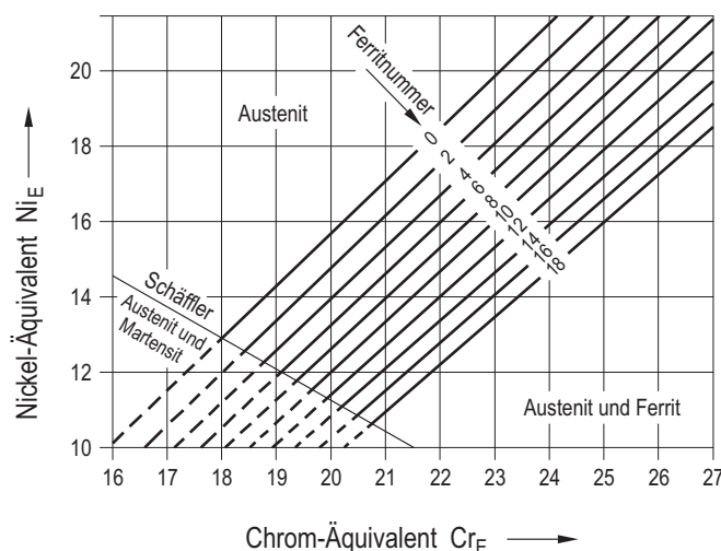
Bild D-1: Zusammenhang zwischen der chemischen Zusammensetzung und den Ferritnummern von aufgeschmolzenem Grundwerkstoff oder Schweißgut (nach W. T. De Long [2])
