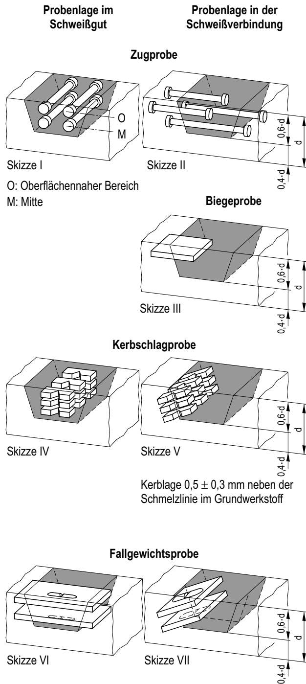
Bild 25-1: Probenentnahme bei Verfahrensprüfungen für Ausmündungsschweißungen
