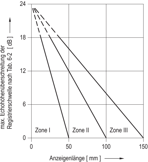
Bild 6-3: Zulässige Anzeigenlängen und Echohöhen bei der Senkrechteinschallung in axialer Richtung (Einschallrichtungen 1 und 2 in Bild 6-2) bei geschmiedeten Platten für Rohrböden
