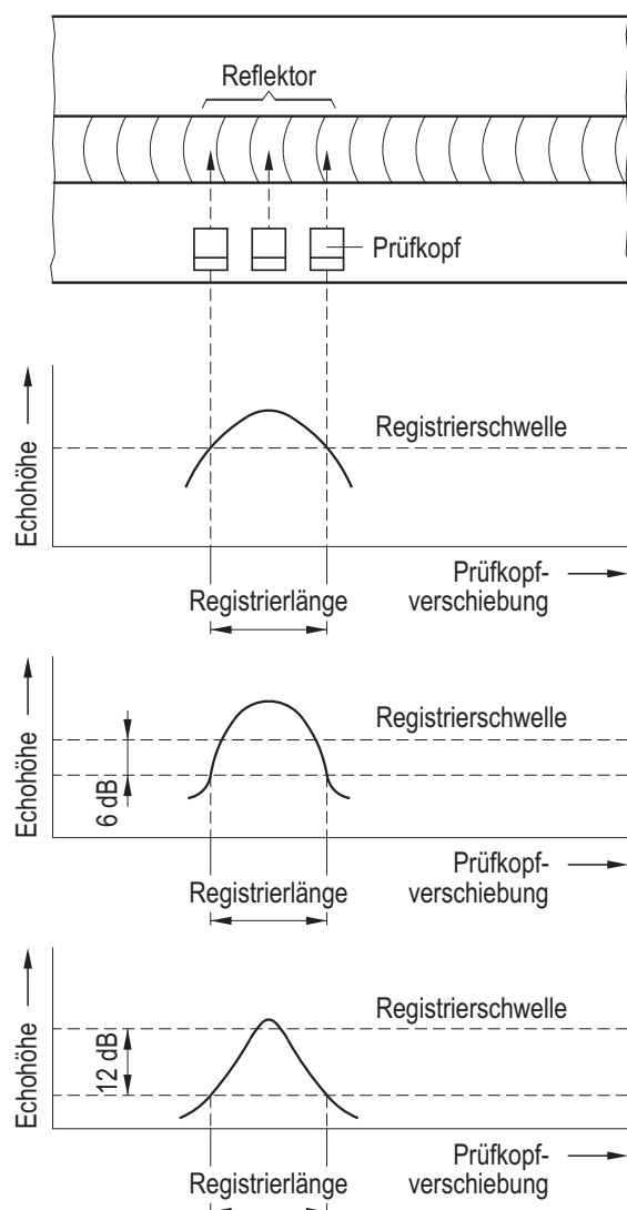
Bild B-20: Bestimmung der Registrierlänge
