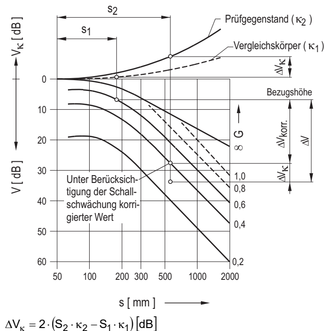
Bild B-8: Berücksichtigung der Schallschwächung im AVG-Diagramm für den Fall \kappa_2 > \kappa_1 (Beispiel)
