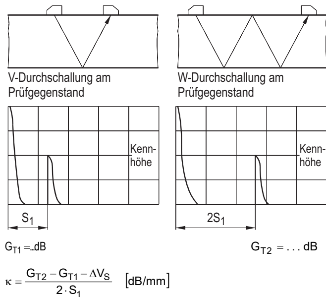
Bild B-7: Bestimmung der Schallschwächung bei der Schrägeinschallung
