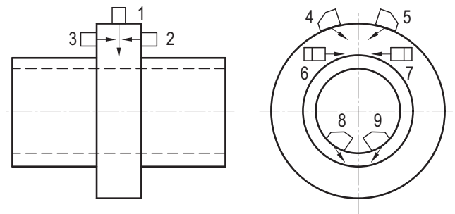
Bild 9-2: Einschallpositionen für den Kragenbereich im Schmiedezustand
