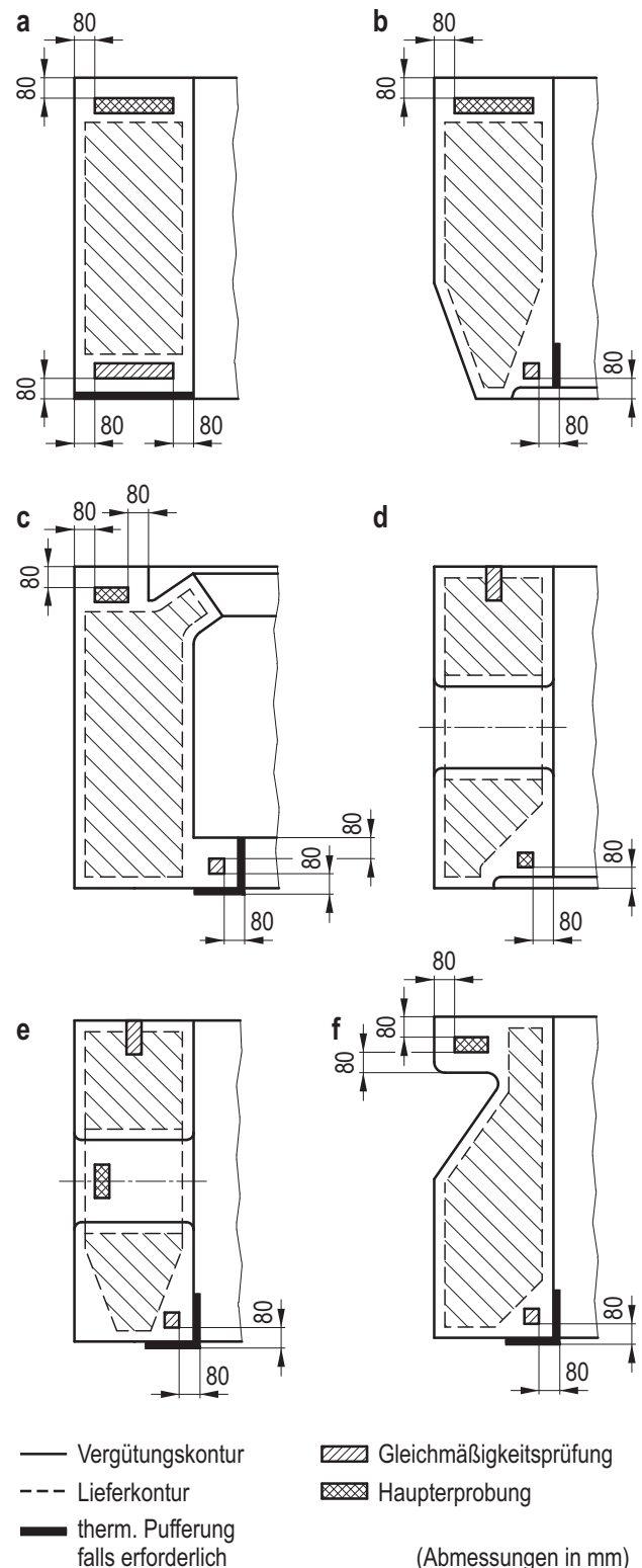
Bild 4-1: Beispiele für Probenentnahmeorte bei Erzeugnissen nach Abschnitt 4.3.1.3
