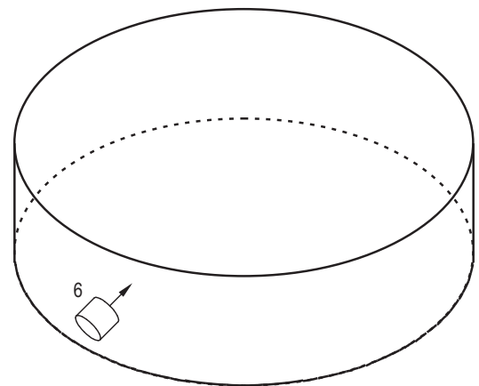
Bild 12-2: Einschallrichtung 6 bei der Ultraschallprüfung
