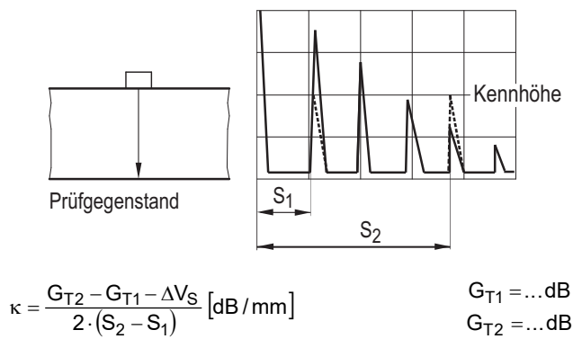
Bild B-6: Bestimmung der Schallschwächung bei der Senkrechteinschallung (Beispiel)
