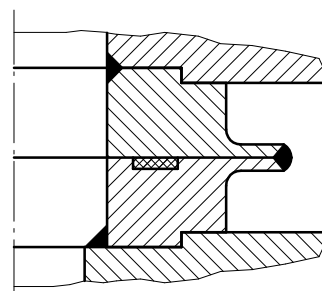
Bild 5.2-2: Beispiele für HV- und DHV-Nähte bei Anschweißungen
