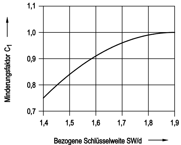
Bild A 2.8-6: Faktor C_1 zur Kennzeichnung der Verminderung der Abstreifigkeit von Bolzen- und Muttergewinde infolge Mutteraufweitung
