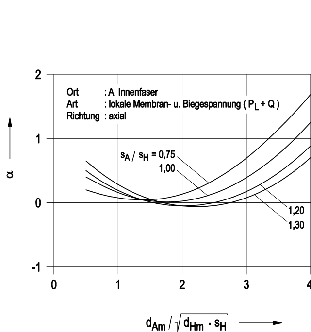
Bild 8.2-8: Spannungsbeiwert \alpha für Stützen in zylindrischer Schale unter Innendruck
