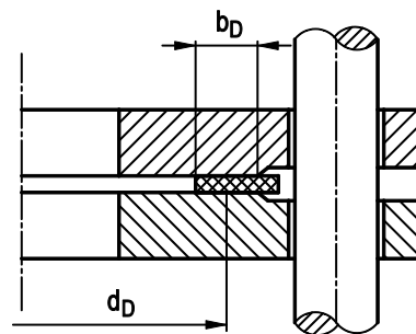
Bild A 2.10-2: Darstellung der Dichtungsbreite b_D
