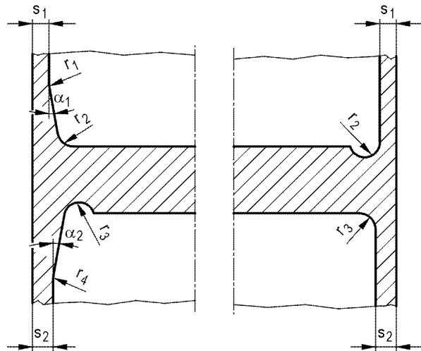
Bild 5.3-1: Beispiele für Rohrboden-Ausführungsformen
