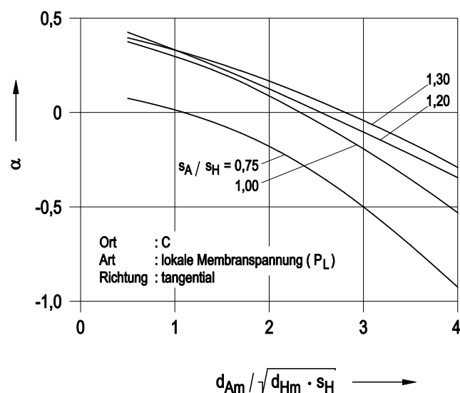
Bild 8.2-7: Spannungsbeiwert \alpha für Stützen in zylindrischer Schale unter Innendruck
