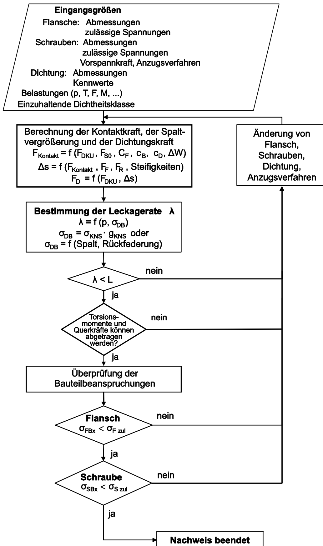
Bild A 2.9-11: Nachweisführung für Flanschverbindungen mit Dichtungen im Kraftnebenschluss (schematisch)
