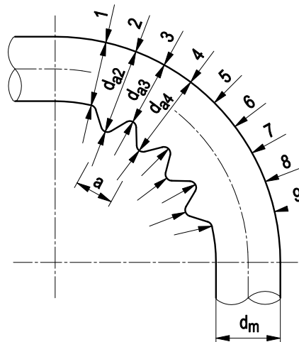
Bild A 4-1: Falten am Rohrbogen
