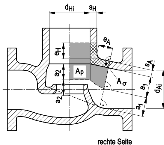
Bild A 3.1-7: Gehäusekörper
