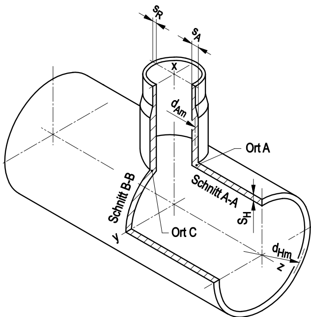
Bild 8.2-1: Stützen an zylindrischer Schale
