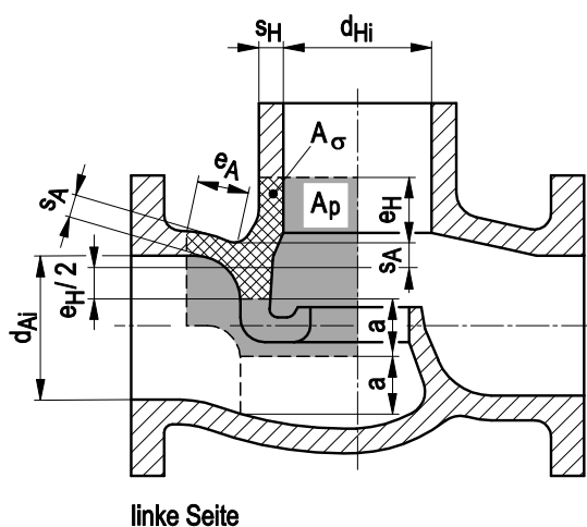
Bild A 3.1-8: Zylindrischer Gehäusekörper
