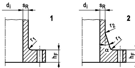
Bild 5.2-7: Vorschweißflansche
