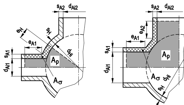
Bild A 3.1-10: Gehäusekörper
