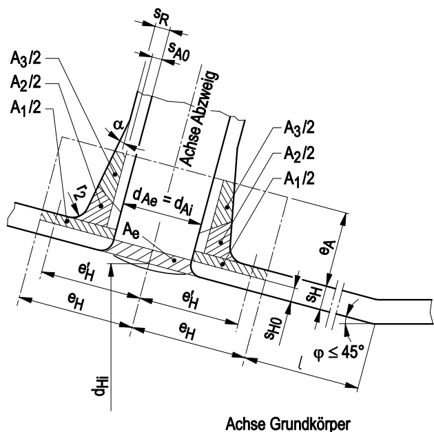
Bild A 2.7-10: Kegelschale mit Ausschnittsverstärkung
