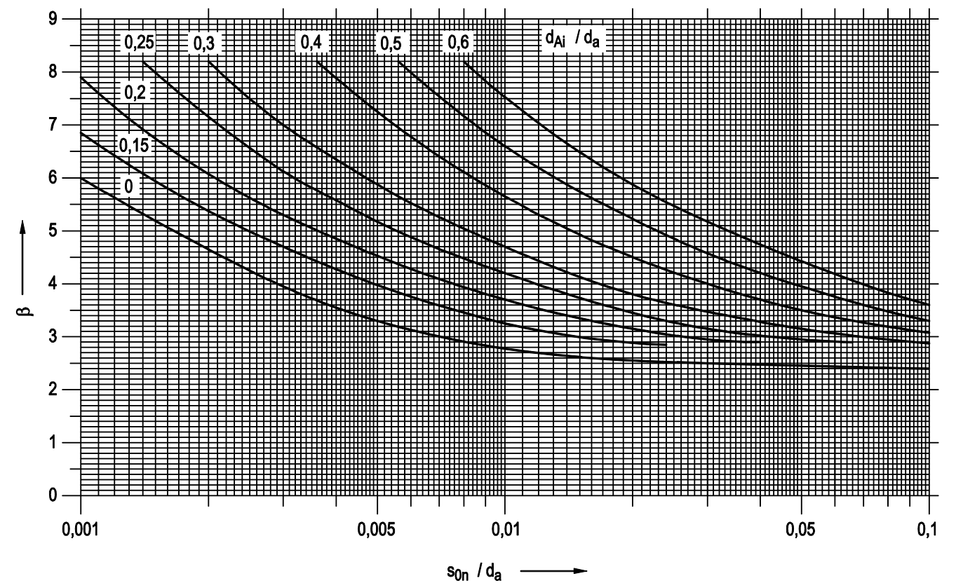
Bild A 2.5-3: Berechnungsbeiwerte \beta für gewölbte Böden in Klöpperform
