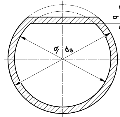
Bild 7.1-2: Abflachung q
