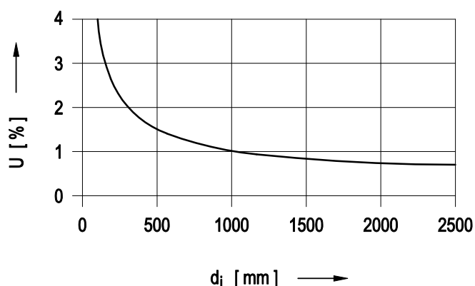
Bild 7.1-4: Unrundheiten
