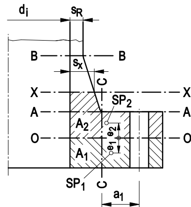
Bild A 2.9-1: Flanschquerschnitt
