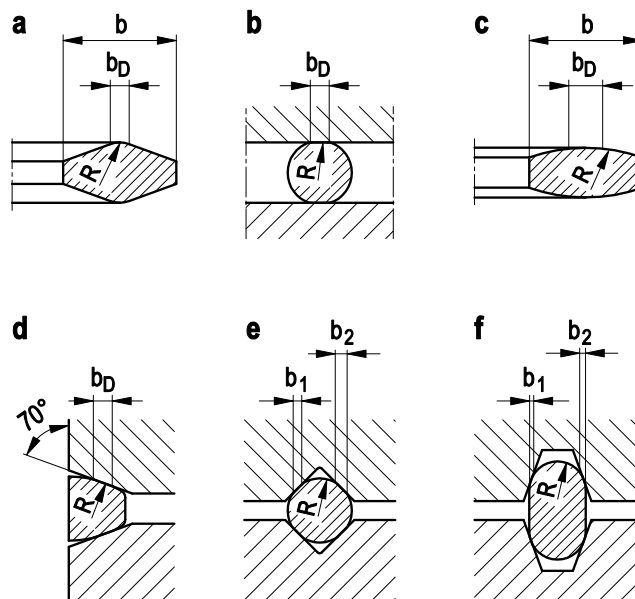
Bild A 2.10-3: Dichtungsprofile für Schmiegedichtungen
