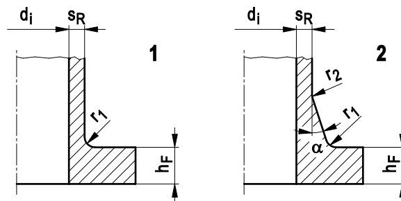
Bild 5.2-6: Vorschweißbunde
