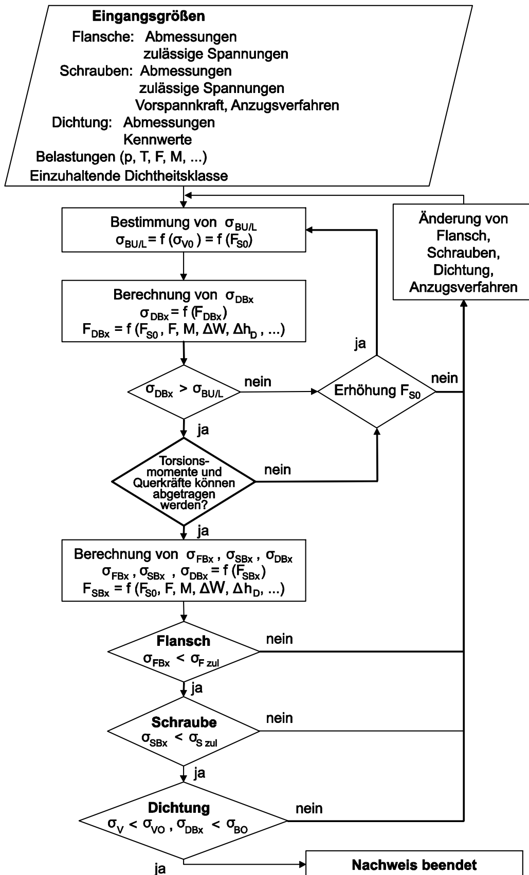
Bild A 2.9-9: Nachweisführung für Flanschverbindungen mit Dichtungen im Krafthaupschluss (schematisch)
