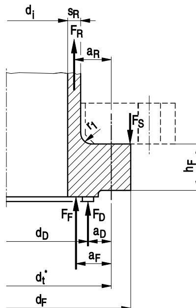
Bild A 2.9-5: Vorschweißbund mit zylindrischem Ansatz
