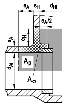
Bild A 3.1-10: Gehäusekörper
