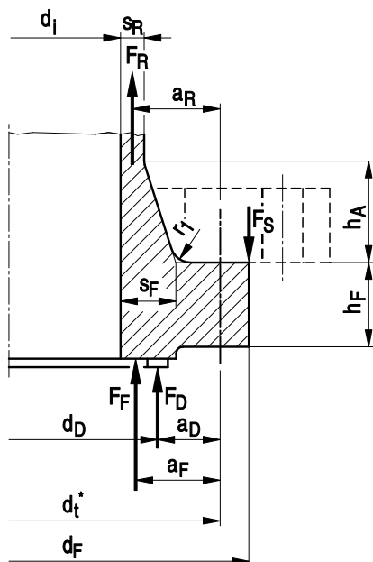
Bild A 2.9-3: Vorschweißbund mit konischem Ansatz
