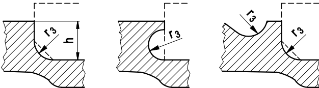
Bild 8.3-3: Zulässige Formen für Ausdehnungen
