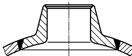
Bild 5.2-8: Beispiele für Stutzen-Ausführungsformen
