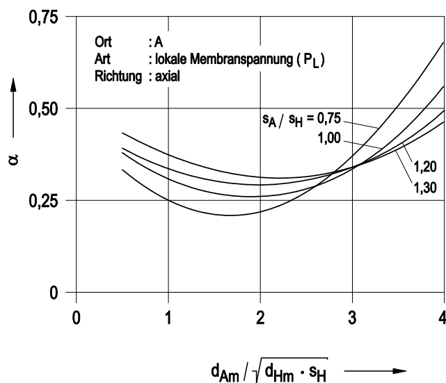
Bild 8.2-6: Spannungsbeiwert \alpha für Stützen in zylindrischer Schale unter Innendruck
