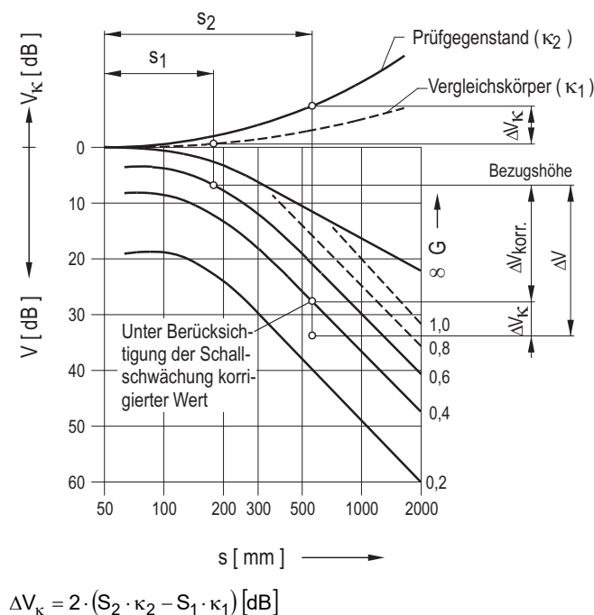
Bild C-8: Berücksichtigung der Schallschwächung im AVG-Diagramm für den Fall \kappa_2 > \kappa_1 (Beispiel)
