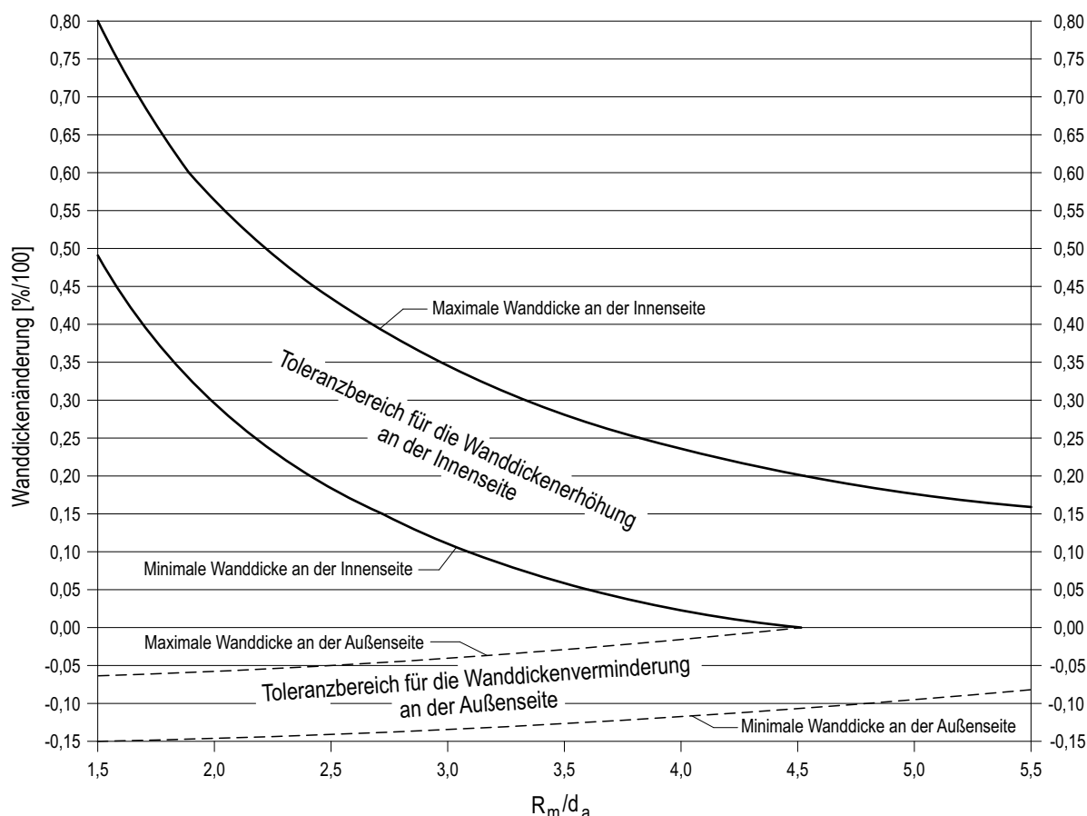
Bild 6-1: Erwartungswerte für die Wanddickenerhöhung an der Krümmungsinnenseite und die Wanddickenverminderung an der Krümmungsaussenseite von Standard-Induktivbiegungen in Abhängigkeit vom Verhältnis R_m/d_a
