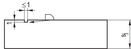
Bild C-11: Vergleichskörper für die Einstellung der Prüfempfindlichkeit bei Anwendung der Kriechwellentechnik (primäre Kriechwelle) zur Prüfung von oberflächennahen Bereichen
