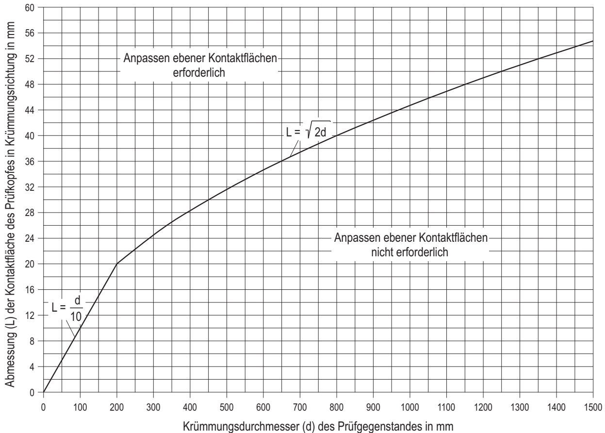
Bild C-1: Anpassbedingungen für ebene Kontaktflächen von Winkelprüfköpfen bei Einschlüsselung in konvexe Kontaktflächen des Prüfgegenstandes
