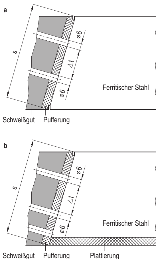
Bild 12-18: Lage der Flachbodenbohrungen und der Nuten für die Prüfung der Grenzfläche zum ferritischen Grundwerkstoff auf Bindung
