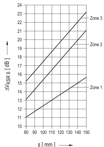
Bild D-3: Prüfbereichsaufteilung für den Wanddickenbereich (mm) 80 \leq s \leq 150 für 2 MHz-Prüfköpfe
