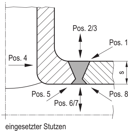
Bild 12-13: Einschallpositionen und Anzahl der Einschallwinkel bei der Stutzenprüfung (aufgesetzter Stutzen) sowie Auswertebereiche der Schrägeinschallung
