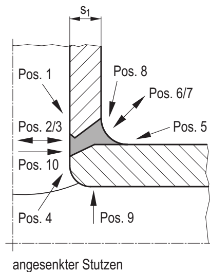
Bild 12-11: Einschalldpositionen und Anzahl der Einschalldwinkel bei der Stützenprüfung (durchgesteckter Stützen) sowie Auswertebereiche der Schrägeinschallung
