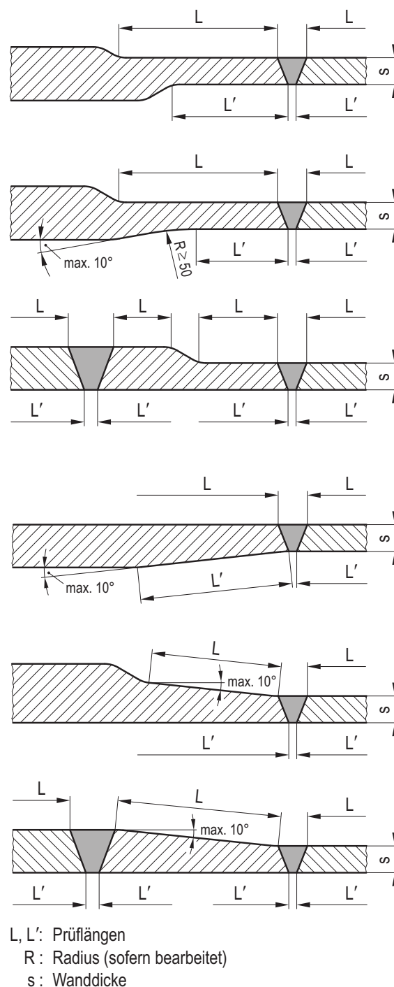
Bild 12-1: Beispiele für die konstruktive Gestaltung von Wanddickenübergängen unter Berücksichtigung der erforderlichen Prüflängen für die Ultraschallprüfung von Stumpfnähten mit \geq DN 80 und s \geq 8 mm
