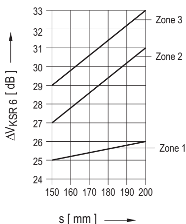
Bild D-13: Prüfbereichsaufteilung für den Wanddickenbereich (mm) 150 \leq s < 200 für 1 MHz-Prüfköpfe
