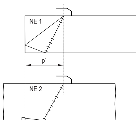
Bild C-15: Schallfeldgeometrien bei der Umwandlung von Transversalwellen
