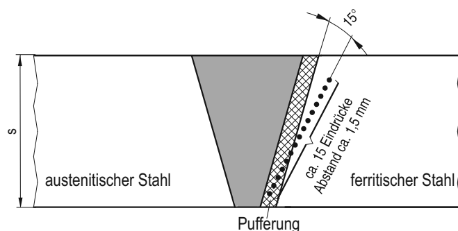
Bild 9-16: Lage der Härtereihe bei der Härteprüfung HV 5 an gepufferten Verbindungsschweißungen zwischen ferritischem und austenitischem Stählen
