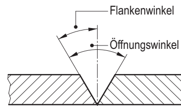
Bild 9-1: Definition des Flanken- und Öffnungswinkels (schematisch)
