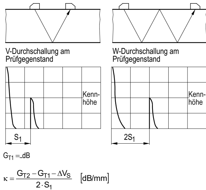
Bild C-7: Bestimmung der Schallschwächung bei der Schrägeinschallung
