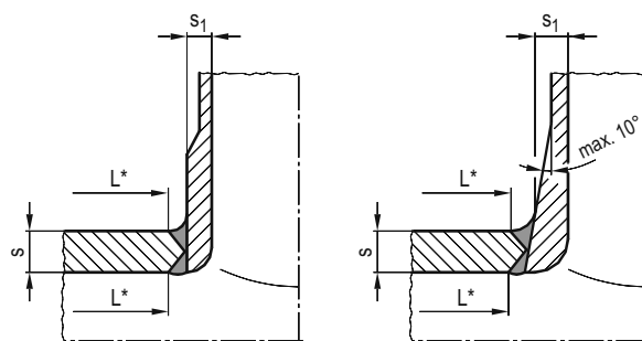
Durchgesteckte Stutzen
