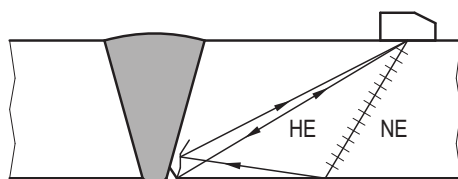
Bild C-16: Prüfung von Komponenten mit Nennwanddicken größer als 8 mm und gleich oder kleiner als 20 mm mittels Longitudinalwellen (Prüfkopf 70 Grad SEL)
