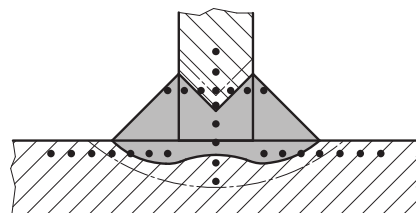
Beispiele für die Lage von Härtereihen
