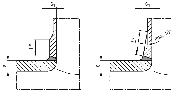
Aufgesetzte Stutzen
