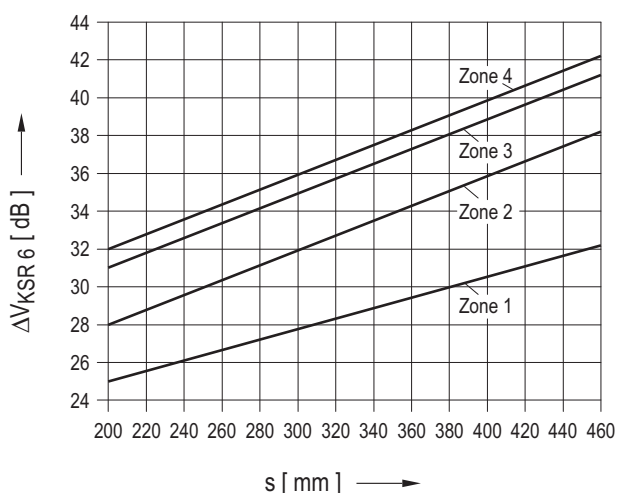
Bild D-15: Prüfbereichsaufteilung für den Wanddickenbereich (mm) 200 \leq s \leq 460 für 1 MHz-Prüfköpfe
