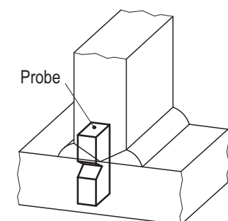
Skizze 4 Kerblage in der WEZ
