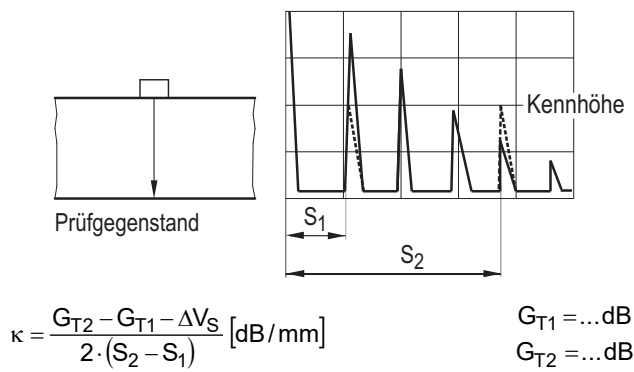
Bild C-6: Bestimmung der Schallschwächung bei der Senkrechteinschallung (Beispiel)
