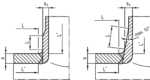
Durchgesteckte Stutzen
