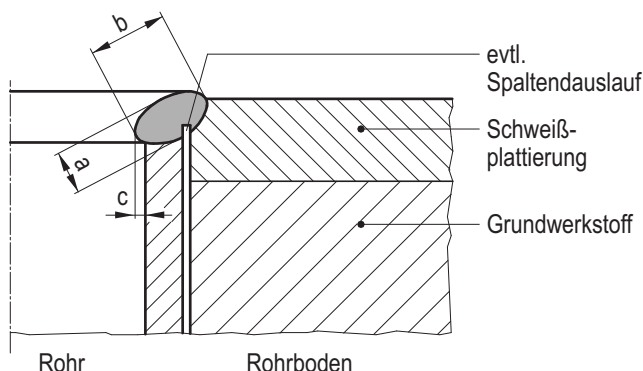
Bild 9-13: Rohreinschweißung in Rohrboden
