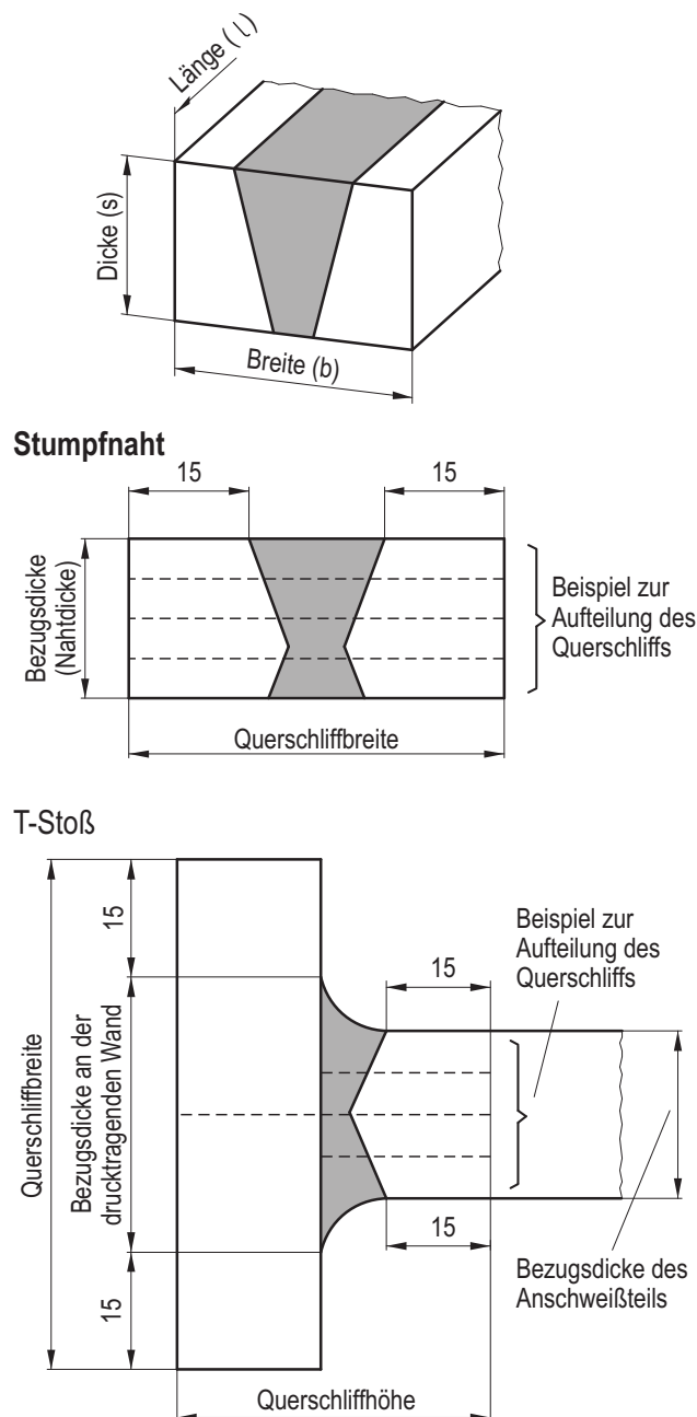
Bild B-1: Probenstücke für erweiterte Querschliffuntersuchungen
