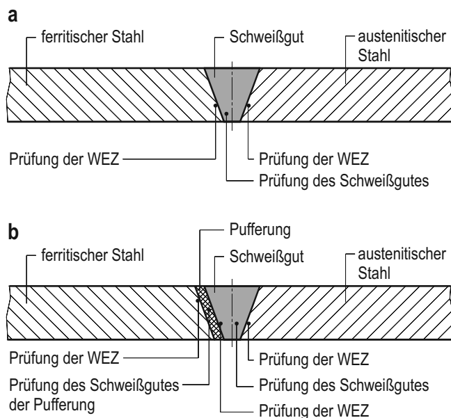
Bild 9-15: Prüfbereiche für Verbindungsschweißungen zwischen ferritischem und austenitischem Stählen
