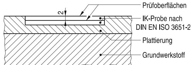
Skizze 1: Korrosionsprüfung
