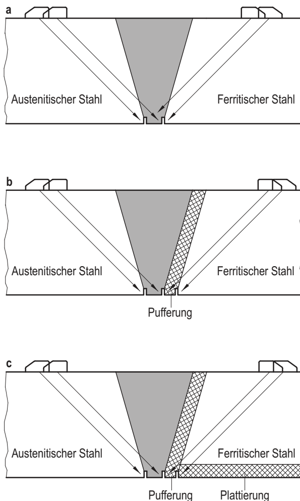
Bild 4-2: Lage der Nuten und Einschallrichtungen für die Längsfehlerprüfung von Schweißverbindungen zwischen ferritischen und austenitischen Stählen
