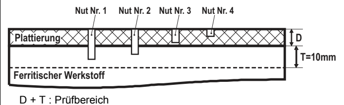
Bild 4-4: Lage der Nuten für die Prüfung plattierter Oberflächen
