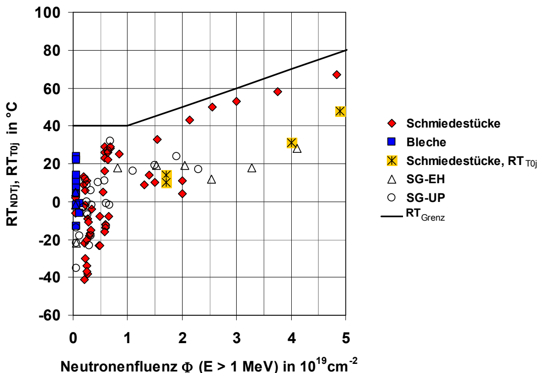
Bild B-1: RT_{\text{NDTj}} , RT_{\text{T0j}} als Funktion der Neutronenfluenz, Grundwerkstoff- und Schweißgutergebnisse der Bestrahlungsüberwachungsprogramme der deutschen RDB (SWR und DWR); nur Schweißgüter mit Massenanteilen \text{Cu} \leq 0,15 \% und 0,05 \% < \text{Ni} \leq 1,7 \% .
