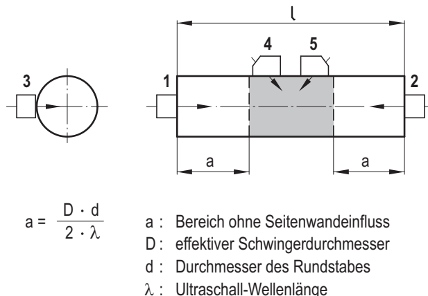
Bild B-1: Einschallpositionen bei Rundstäben
