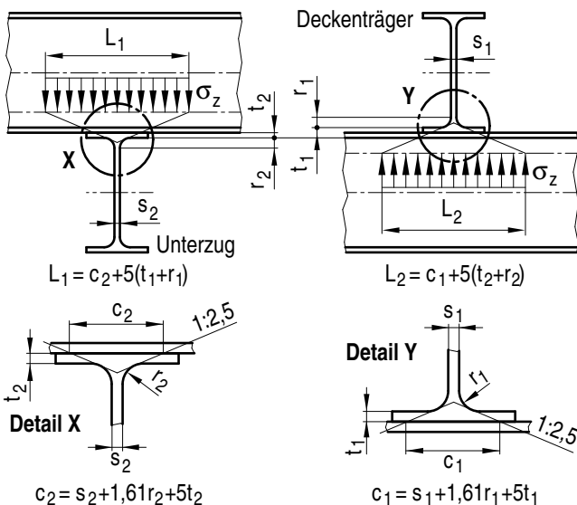
Bild 4-2: Steifenlose Lasteinleitung bei Walzprofilen mit H-Querschnitt (angelehnt an DIN 18800-1 historisch)
