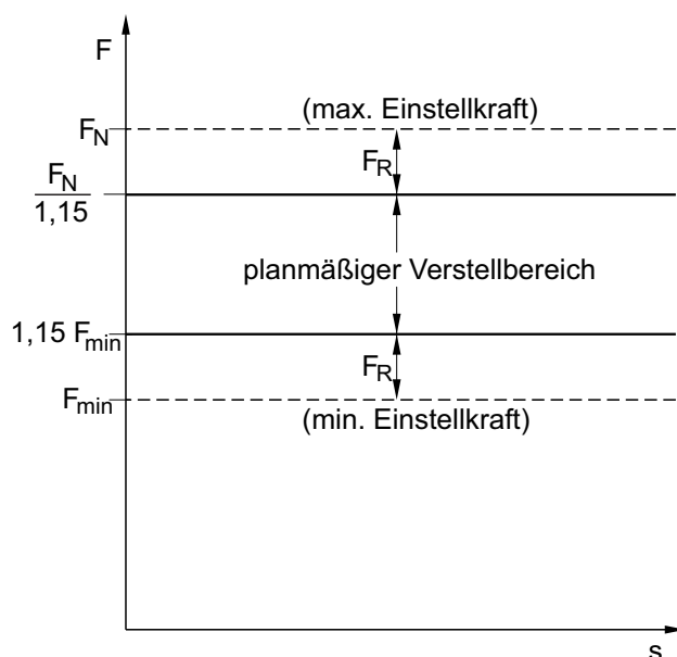
Bild C 2-2: Verstellbereich Konstanthänger
