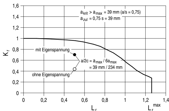
Bild D 2-13: Ermittlung der zulässigen Risstiefe
