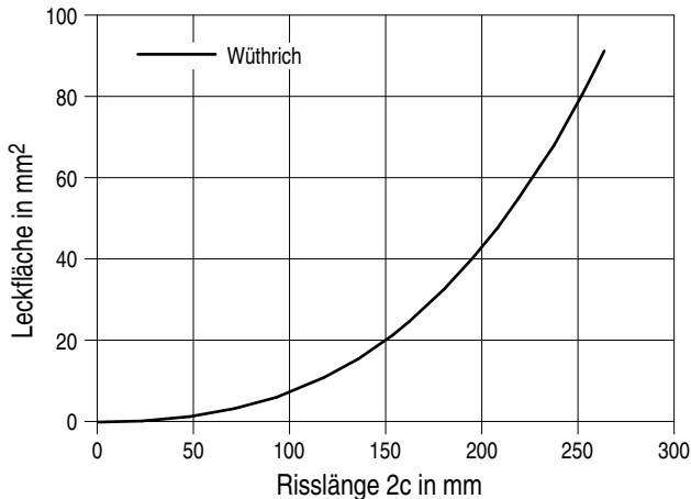
Bild D 1-16: Leckfläche in Abhängigkeit von der Risslänge 2c für die betrachtete austenitische Rohrleitung mit Umfangsris
