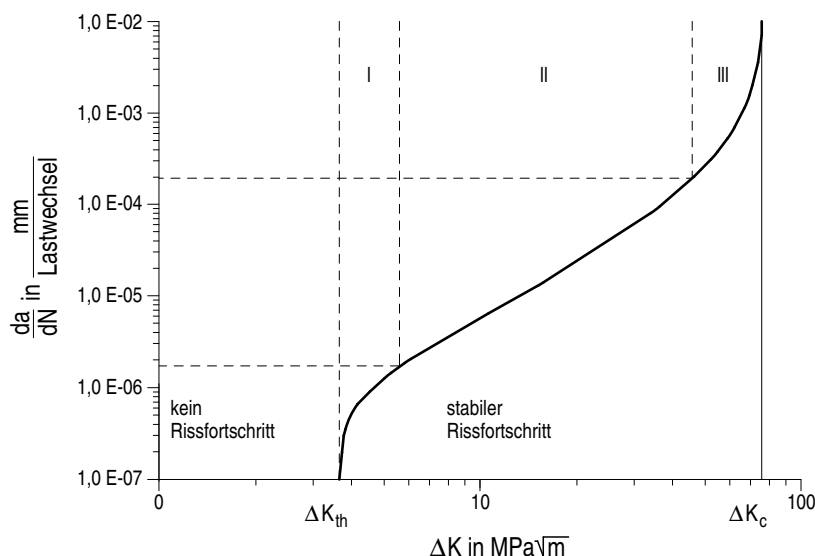
Bild B 2.5-1: Rissfortschritt bei zyklischer Beanspruchung, Prinzipdarstellung [35]
