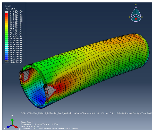
Bild D 1-10: Axialspannungsverteilung
