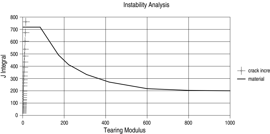
Bild D 2-8: Instabilitätsanalyse für Innendruck
