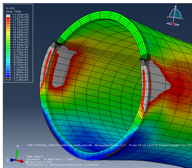
Bild D 1-9: Finite Element Modell und Randbedingungen (Durchriss im Bereich des Anschlusses eines Rohrs an eine Komponente; alle Freiheitsgrade im gesamten Ligament fixiert, wodurch die Leckfläche gegenüber anderen Einspannbedingungen minimiert wird)
