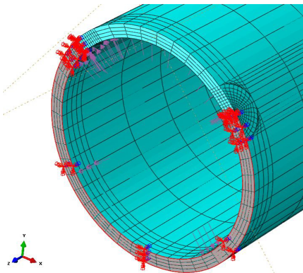
Bild D 1-9: Finite Element Modell und Randbedingungen (Durchriss im Bereich des Anschlusses eines Rohrs an eine Komponente; alle Freiheitsgrade im gesamten Ligament fixiert, wodurch die Leckfläche gegenüber anderen Einspannbedingungen minimiert wird)
