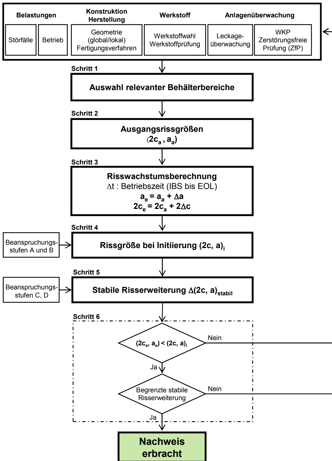
Bild A-5: Bruchmechanische Analyse von postulierten Rissen in Behältern
