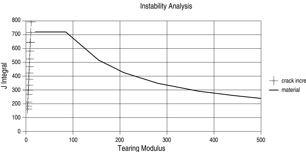
Bild D 2-9: Instabilitätsanalyse für Biegung + Innendruck
