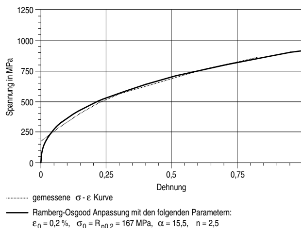
Bild B 2.2-5: Wahre Spannungs-Dehnungs-Kurve (schematisch)
