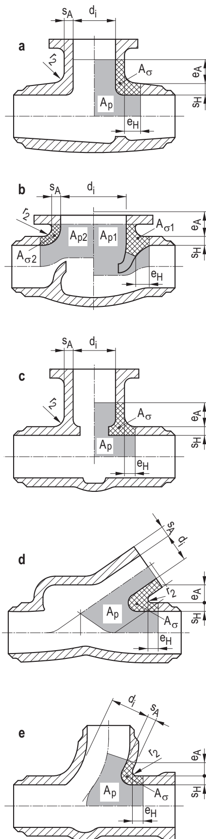
Bild 8.4-1: Flächenvergleichsmethode
