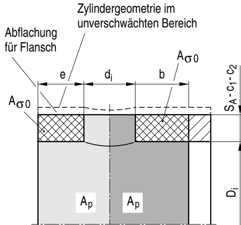
Bild A 3.3-5: Berechnungsschema für Rohrgehäuse mit Abflachung und Ausschnitt
