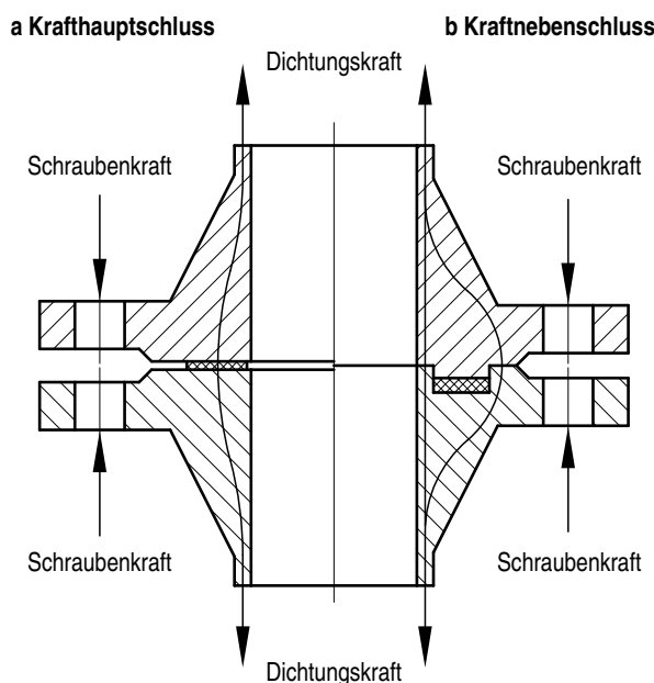
Bild A 2.9-1: Darstellung einer Flanschverbindung mit der Dichtung im KHS und im KNS (schematisch)
