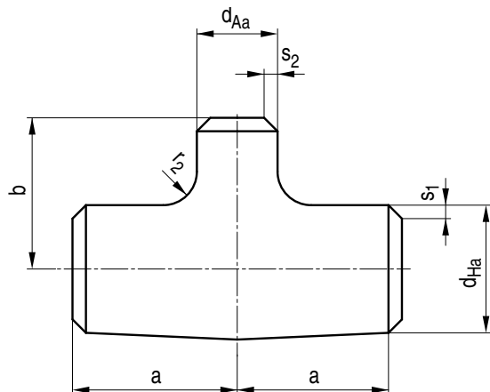
Bild A 5-8: Gepresstes Einschweiß-T-Stück
