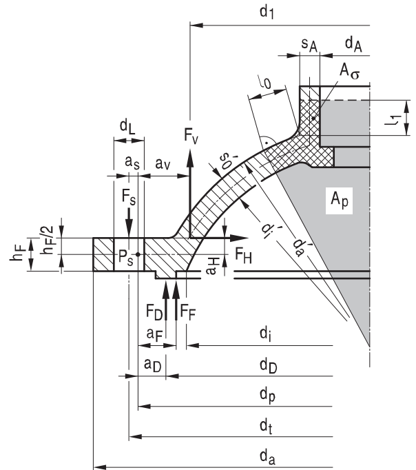
Bild A 2.6-2: Tellerboden mit tiefgewölbter Kugelschale (Ausführung II, y = 0 )
