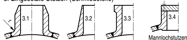
Bild 5.2-6: Beispiele von Stutzen-Ausführungsformen
