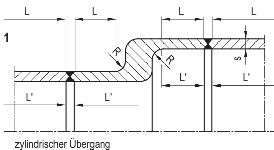
Bild 5.2-4: Ausführungsformen von Schweißnähten an Stutzen
