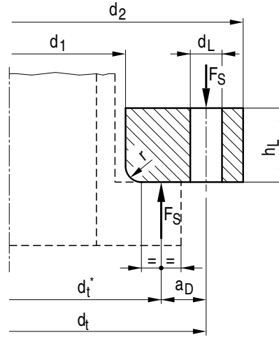
Bild A 2.10-6: Losflansch
