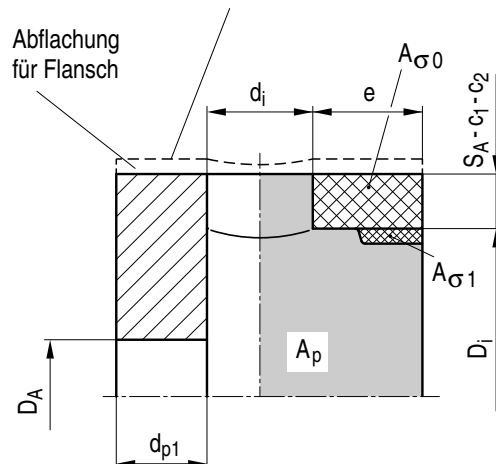
Bild A 3.3-3: Berechnungsschema für Ringraumgehäuse mit Abflachung und Ausschnitt
