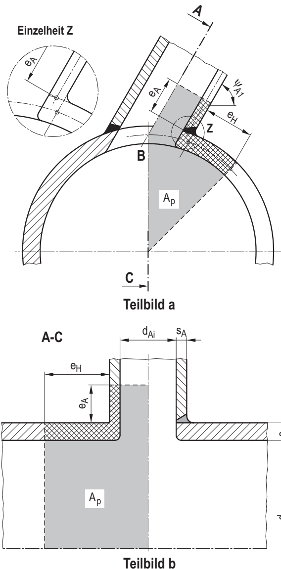
Bild A 5-18: Beanspruchungsschema für eine Zylinderschale mit einem nicht radial angeordneten Abzweig
