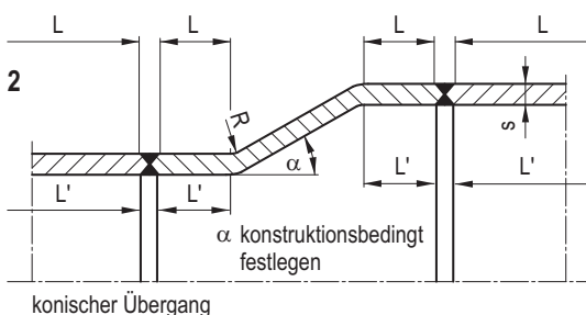
konischer Übergang
