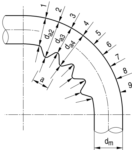
Bild A 5-1: Falten am Rohrbogen
