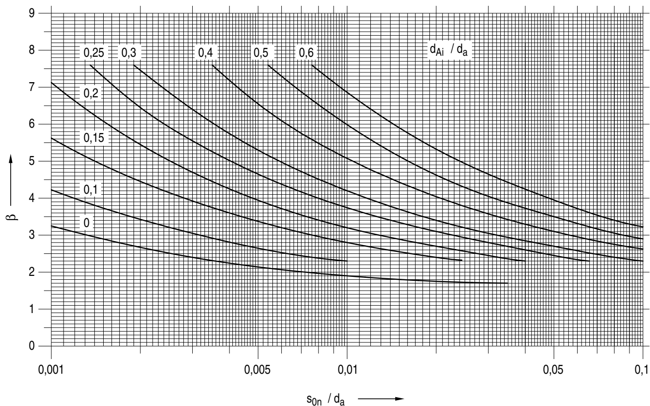
Bild A 2.5-5: Berechnungsbeiwerte \beta für gewölbte Böden in Korbbogenform
