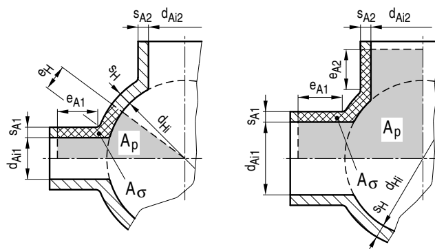
Bild A 4.1-10: Gehäusekörper
