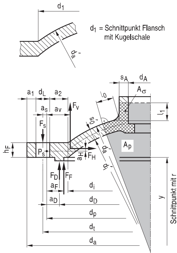
Bild A 2.6-1: Tellerboden mit flachgewölbter Kugelschale (Ausführung I, y > 0 )
