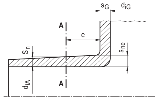
Bild 8.4-5: Maßgebender Schnitt an konischen Armaturengehäusen
