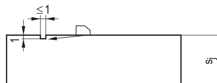
Bild D-11: Vergleichskörper für die Einstellung der Prüfempfindlichkeit bei Anwendung der Kriechwellentechnik (primäre Kriechwelle) zur Prüfung von oberflächennahen Bereichen
