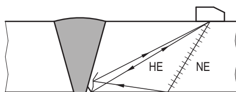
Bild D-16: Prüfung von Komponenten mit Nennwanddicken größer als 8 mm und gleich oder kleiner als 20 mm mittels Longitudinalwellen (Prüfkopf 70 Grad SEL)
