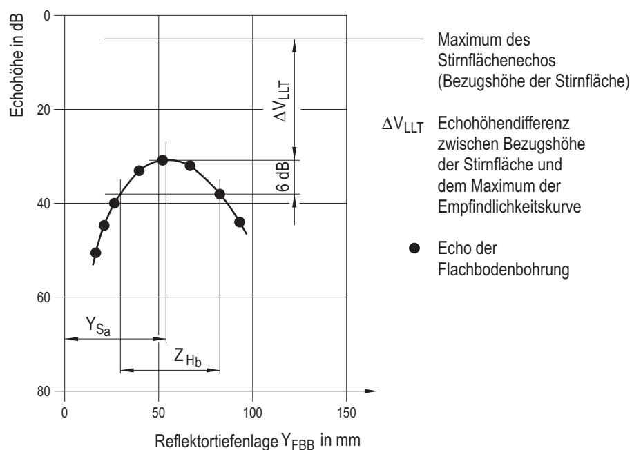
Bild D-18: Beispiel für ein LLT-Empfindlichkeitsdiagramm
