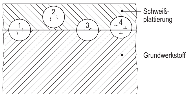
Bild 8-10: Probenlagen und Prüforte an Prüfstücken mit Auftragschweißungen
