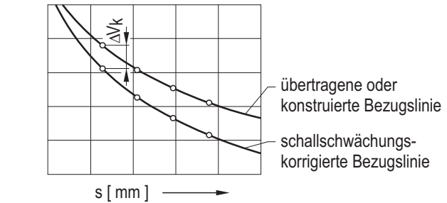
Bild D-9: Berücksichtigung der Schallschwächung bei der Bezugslinien-Methode für den Fall \kappa_2 > \kappa_1 (Beispiel)
