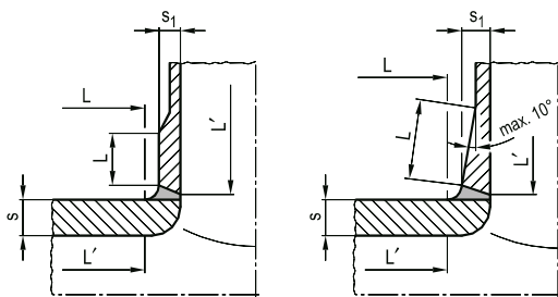
Durchgesteckte Stutzen
