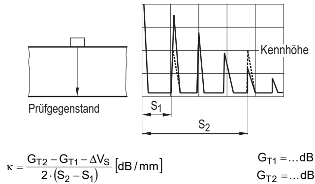
Bild D-6: Bestimmung der Schallschwächung bei der Senkrechteinschallung (Beispiel)
