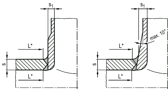
Durchgesteckte Stutzen
