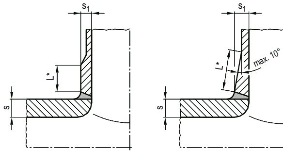
Aufgesetzte Stutzen
