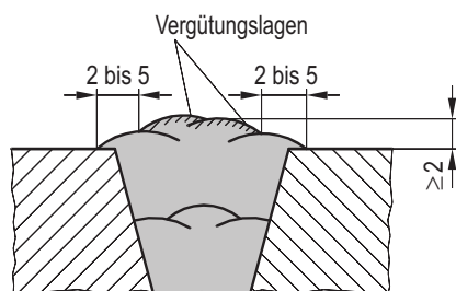
Bild 5-1: Vergütungsagententechnik ferritischer Schweißnähte am Beispiel der Schweißposition Wannenlage (PA)
