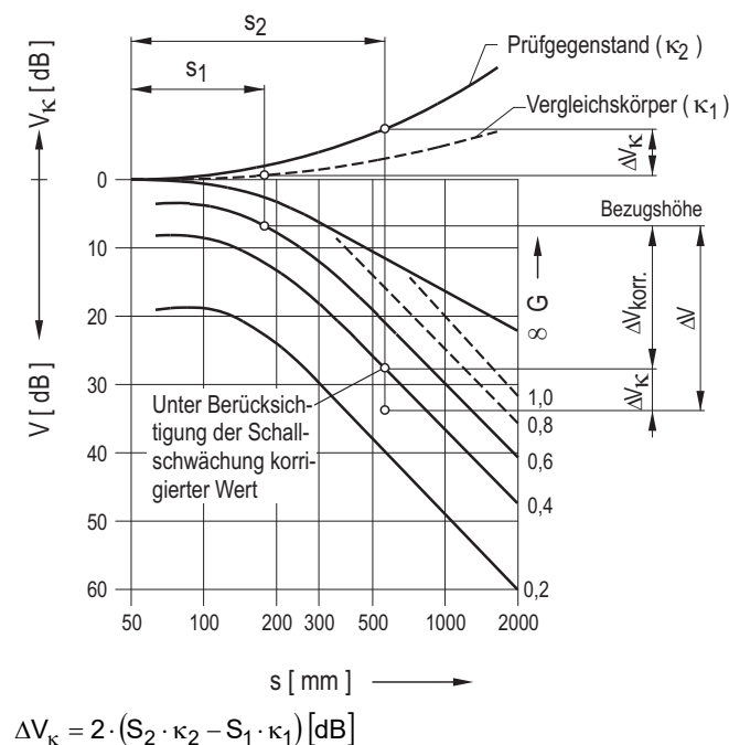
Bild D-8: Berücksichtigung der Schallschwächung im AVG-Diagramm für den Fall \kappa_2 > \kappa_1 (Beispiel)
