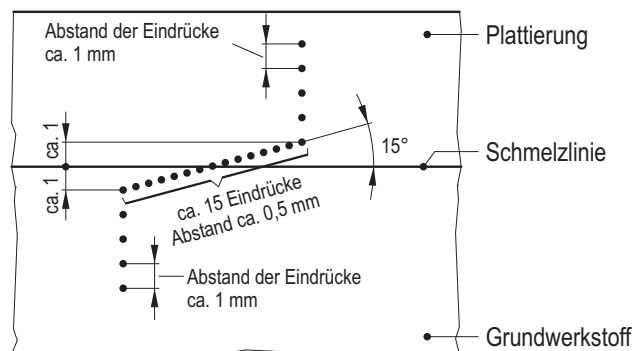
Skizze 2: Härteprüfung
