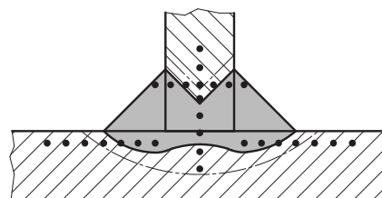
Beispiele für die Lage von Härtereihen
