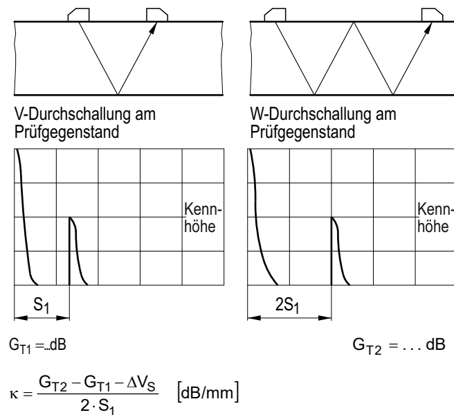
Bild D-7: Bestimmung der Schallschwächung bei der Schrägeinschallung
