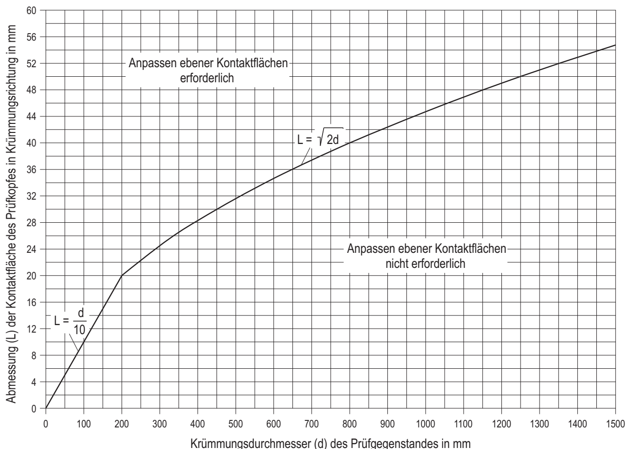
Bild D-1: Anpassbedingungen für ebene Kontaktflächen von Winkelprüfköpfen bei Einschließung in konvexe Kontaktflächen des Prüfgegenstandes
