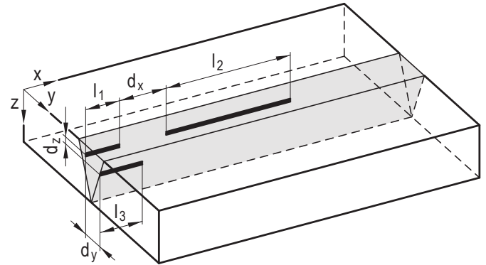
Bild 11-7: Geometrische Anordnung von gehäuften Anzeigen bei der Längsfehlerprüfung
