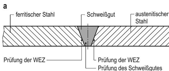
Bild 8-6: Lage der Härtereihe bei der Härteprüfung HV 5 an Querschliffen von ferritischen Verbindungsschweißungen
