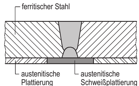
Bild 5-2: Verbindungsschweißung plattierter Bauteile
