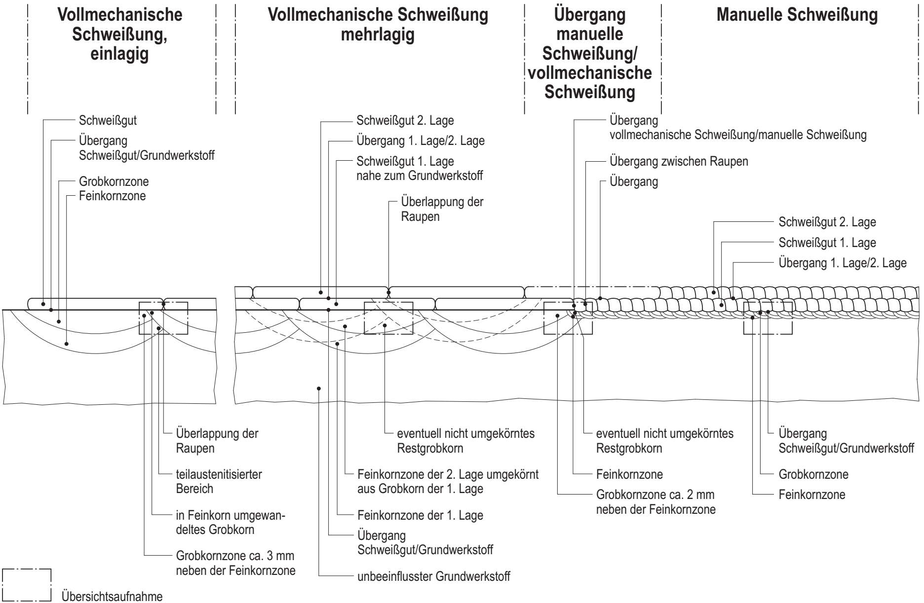
Bild 8-9: Probenlagen und Prüforte an schweißplattierten Prüfstücken (Fortsetzung)
