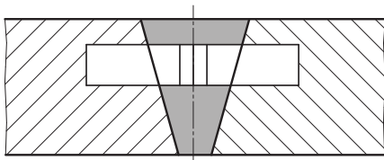
Skizze 1: Lage der Kerbschlagprobe im Schweißgut
