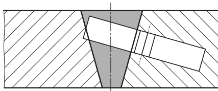
Skizze 2: Lage der Kerbschlagprobe in der Wärmeeinflusszone
