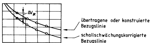
Bild B-8: Berücksichtigung der Schallschwächung im AVG-Diagramm für den Fall \kappa_2 > \kappa_1
