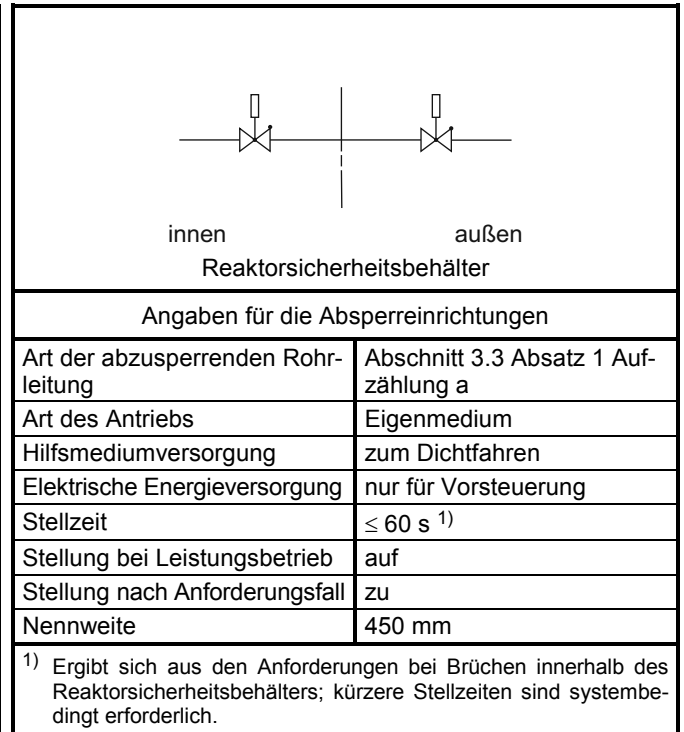
Bild A-3: Beispiel einer Anordnung von Absperreinrichtungen für das Hauptspeisewassersystem beim Siedewasserreaktor
