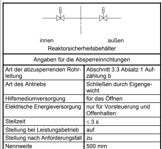
Bild A-4: Beispiel einer Anordnung von Absperreinrichtungen für die Lüftungstechnische Anlage (Unterdruckhaltung) beim Druckwasserreaktor
