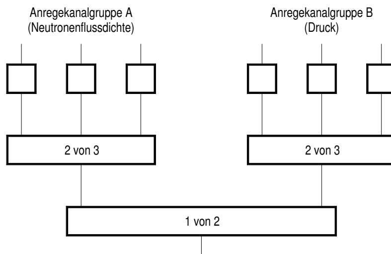
Bild 4-2: Für die Auslösung der Reaktorschnellabschaltung aufgrund von Reaktivitätsstörungen, bei denen zwei aus verschiedenen Prozessvariablen, z. B. Neutronenflussdichte und Druck, abgeleitete Auslösekriterien vorhanden sind und Folgefehler im Bereich der Messwerterfassung ausgeschlossen werden können, ist der hier prinzipiell dargestellte Schaltungsaufbau möglich.
