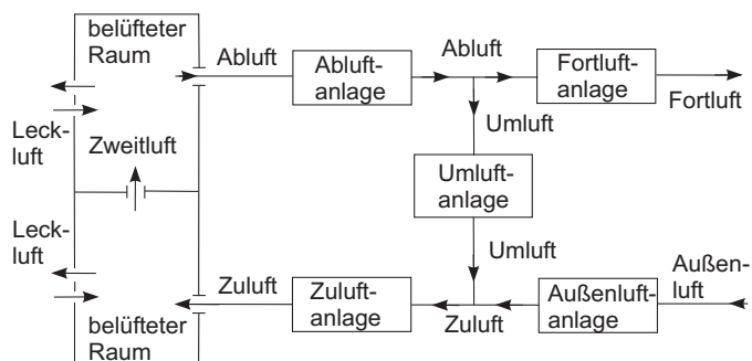
Bild 2-1: Benennungen von Luftströmen und Anlagen
