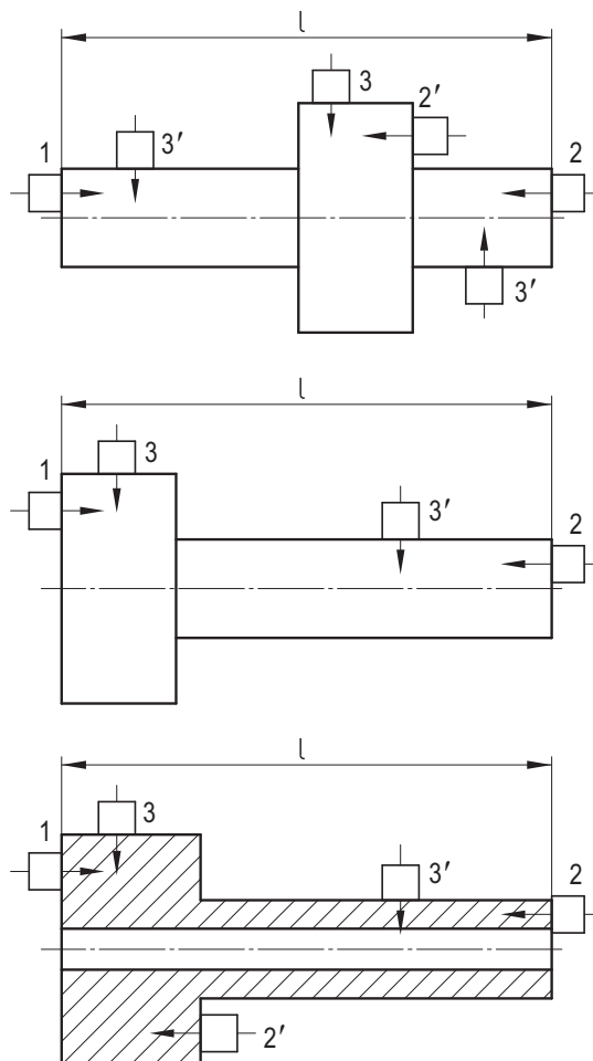
Bild B-6: Einschallpositionen bei Wellen und Achsen mit Absätzen (Beispiele)
