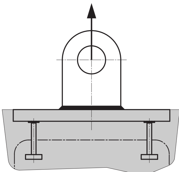
Bild C-7: Tragöse (an einer im Beton verankerten Ankerplatte mit bauaufsichtlicher Zulassung angeschweißt)
