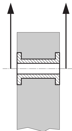
Bild C-8: Im Beton verankerte und verstärkte Durchstecköffnung für einen Bolzen
